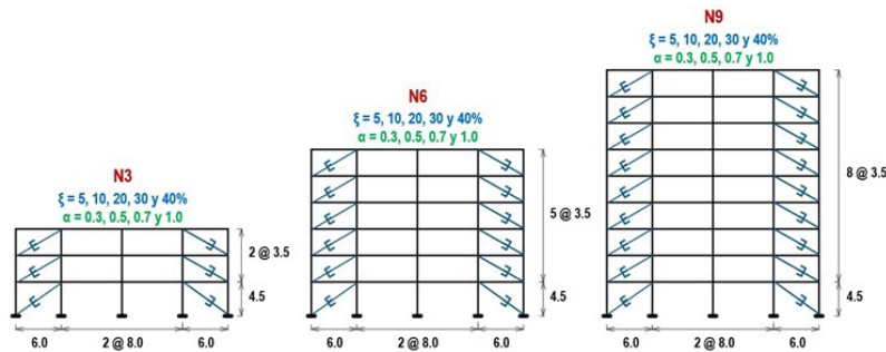
Figura 1 Esquema básico de los prototipos de tres, seis y nueve pisos a evaluar
