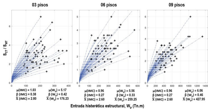
Figura 5 Curvas IDA para los prototipos sin amortiguadores
